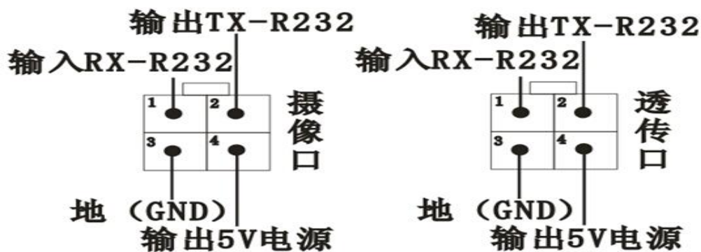
摄像及透传口 (R232) 接口定义
